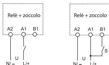
Schema di collegamento (senza START esterno)
