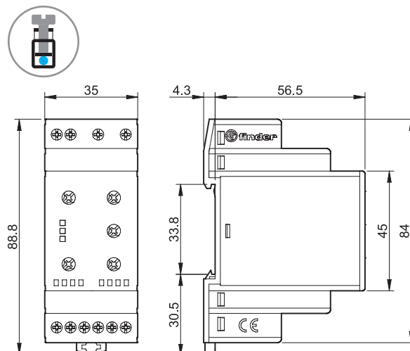
Tipo 70.42 Morsetti a bussola
