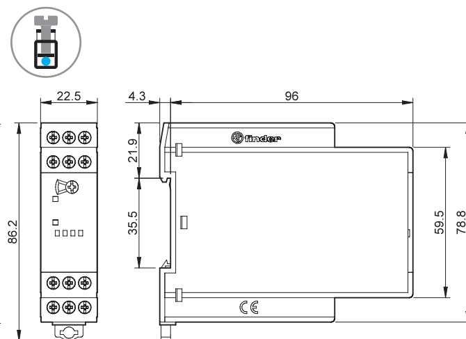
Tipo 70.92 Morsetti a bussola
