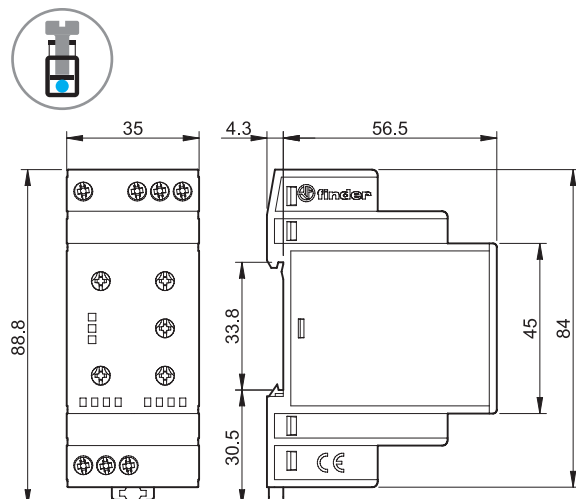
Tipo 70.41 Morsetti a bussola
