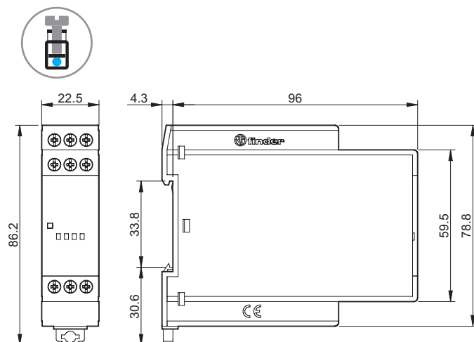
Tipo 70.62 Morsetti a bussola
