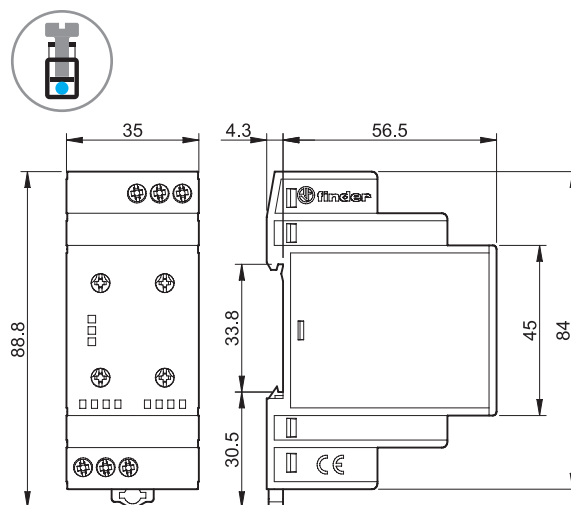
Tipo 70.31 Morsetti a bussola
