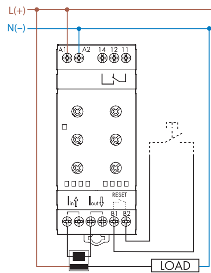
70.51 con collegamento TA
