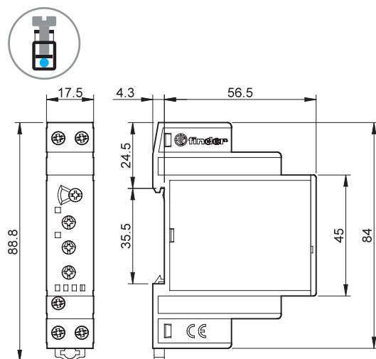
Tipo 70.11 Morsetti a bussola
