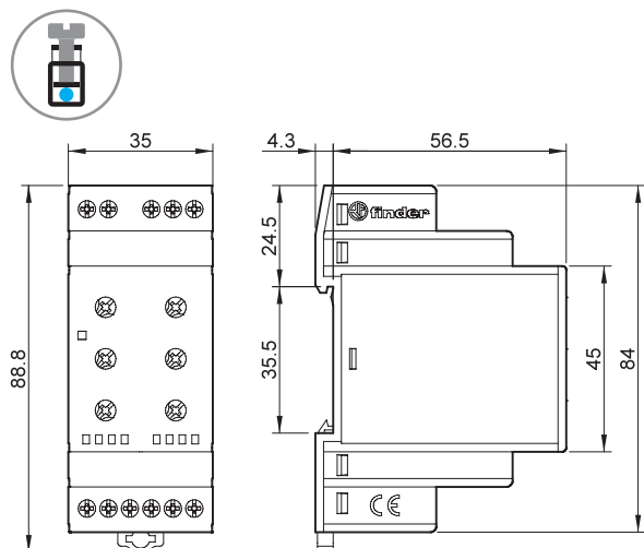
Tipo 70.61 Morsetti a bussola
