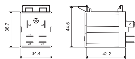
065.08 con relè
