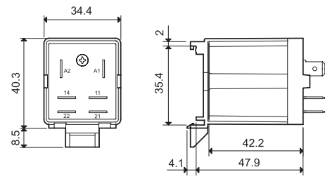
065.07 con relè
