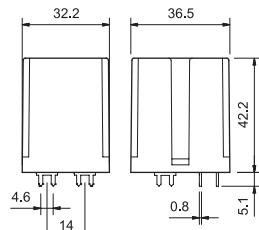
Tipo 65.61
