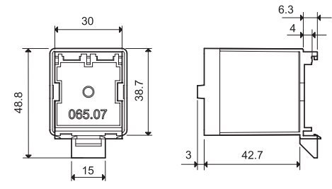
065.07
