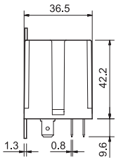
Tipo 65.31
