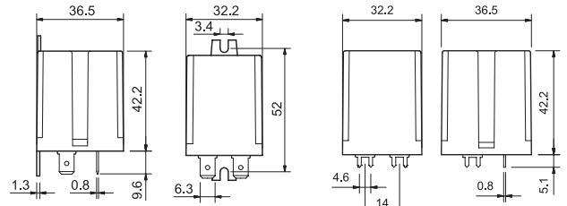
Tipo 65.31- 4300
