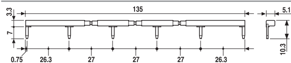
Pettine a 6 poli per tipo 58.P3 e 58.P4
