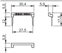
Pettine a 2 poli per tipo 58.P3 e 58.P4
