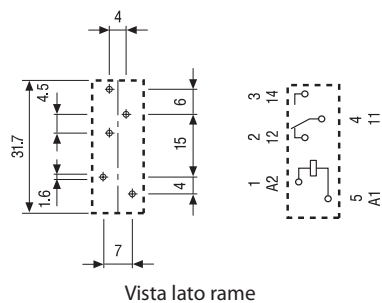
Vista lato rame
