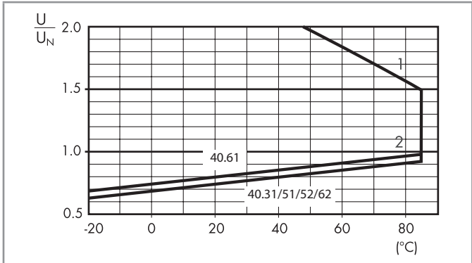
R 40 - Campo di funzionamento bobina DC in funzione della temperatura ambiente Bobina sensibile, tipi 40.31/51/52/61/62
