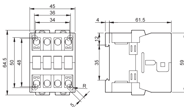
Tipo 6K.13-4350/4374 Morsetti a bussola
