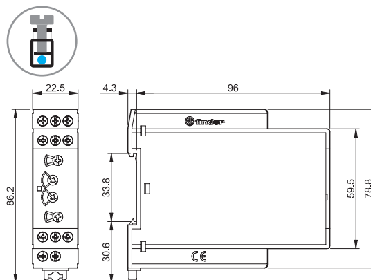
Tipo 83.21 Morsetti a vite
