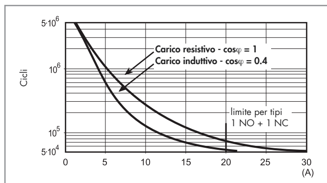
F 65 - Durata elettrica (AC) in funzione della corrente
