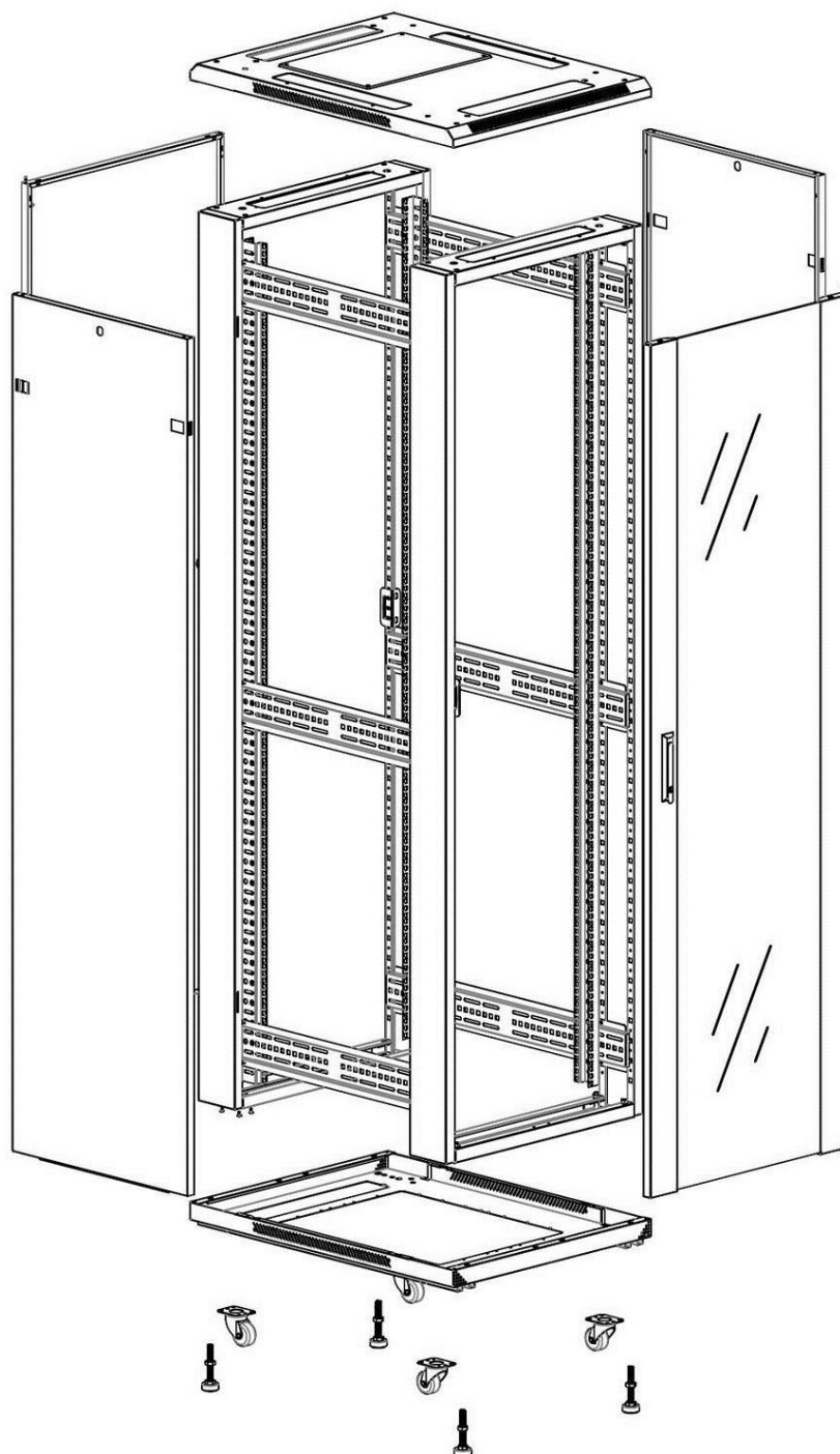
Disegno esploso
