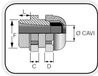
disegno dimensionale / reference details
