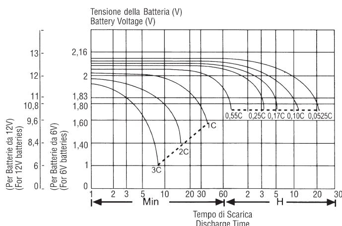
FIG.10 Tensione di fine scarica in funzione della corrente. Discharge current and final discharge voltage.
