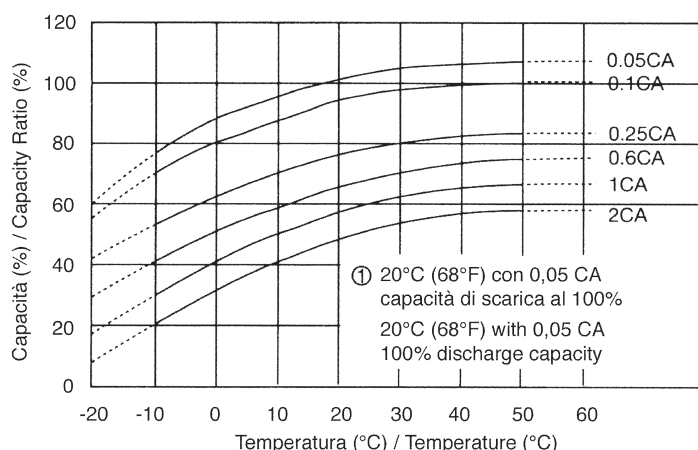
FIG.9 Rendimento delle batterie in funzione della temperatura media di lavoro. Temperature and discharge capacity.
