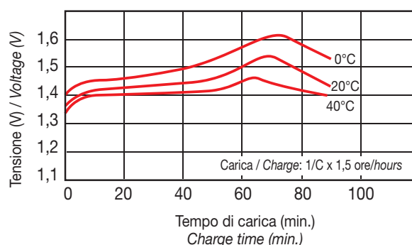
Fig. 5 Effetto della temperatura sulla carica rapida Effect of temperature on rapid charge
