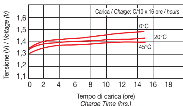
Fig. 3 Effetto della temperatura sulla carica normale Effect of temperature on standard charge
