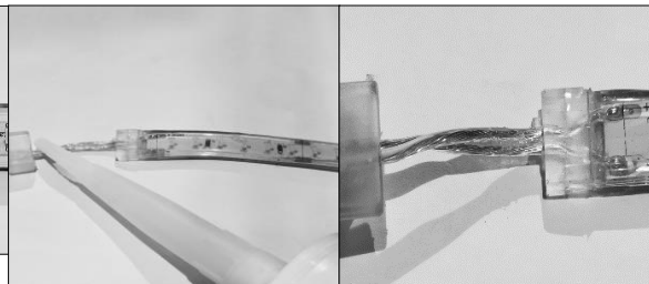
Figura 5a, 5b e 5c. Identificare la sezione di taglio più vicina alla lunghezza desiderata, inserimento tappo di chiusura e aggiunta di silicone per ripristinare il grado IP della striscia LED. NB: Riempire il tappo e la striscia LED di silicone o pasta siliconica specifica per circuiti stampati
