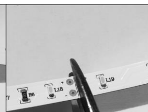
Figura 3b. Sezione di taglio di una striscia LED
