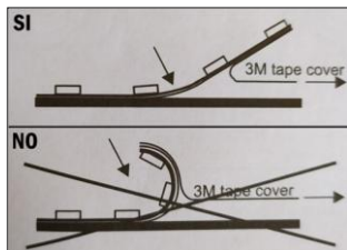
Figura 2. Applicazione della striscia LED con pressione costante e senza torsioni o curvature del circuito stampato
