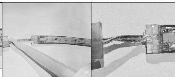
Figura 5a, 5b e 5c. Identificare la sezione di taglio più vicina alla lunghezza desiderata, inserimento tappo di chiusura e aggiunta di silicone per ripristinare il grado IP della striscia LED. NB: Riempire il tappo e la striscia LED di silicone o pasta siliconica specifica per circuiti stampati
