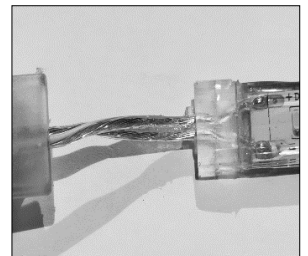
Figura 5a, 5b e 5c. Identificare la sezione di taglio più vicina alla lunghezza desiderata, inserimento tappo di chiusura e aggiunta di silicone per ripristinare il grado IP della striscia LED. NB: Riempire il tappo e la striscia LED di silicone o pasta siliconica specifica per circuiti stampati
