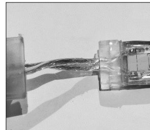
Figura 5a, 5b e 5c. Identificare la sezione di taglio più vicina alla lunghezza desiderata, inserimento tappo di chiusura e aggiunta di silicone per ripristinare il grado IP della striscia LED. NB: Riempire il tappo e la striscia LED di silicone o pasta siliconica specifica per circuiti stampati
