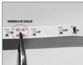
Figura 3a. Sezione di taglio di una striscia LED
