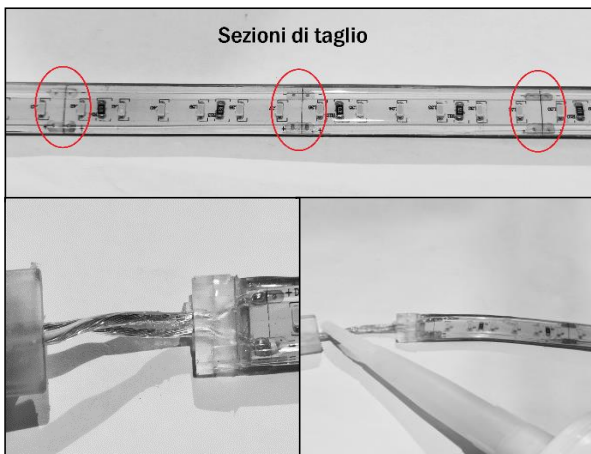
Figura 5a, 5b e 5c. Identificare la sezione di taglio più vicina alla lunghezza desiderata, inserimento tappo di chiusura e aggiunta di silicone per ripristinare il grado IP della striscia LED.
