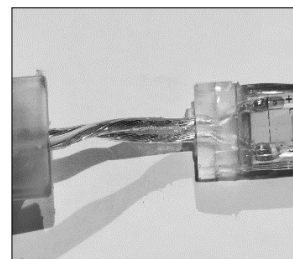
Figura 5a, 5b e 5c. Identificare la sezione di taglio più vicina alla lunghezza desiderata, inserimento tappo di chiusura e aggiunta di silicone per ripristinare il grado IP della striscia LED. NB: Riempire il tappo e la striscia LED di silicone o pasta siliconica specifica per circuiti stampati
