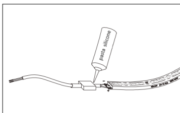
Figura 6. Inserire il tappo di alimentazione riempito di pasta siliconica
