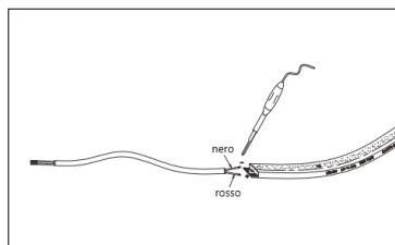
Figura 5. Saldatura del cavo. Utilizzare stagno senza piombo
