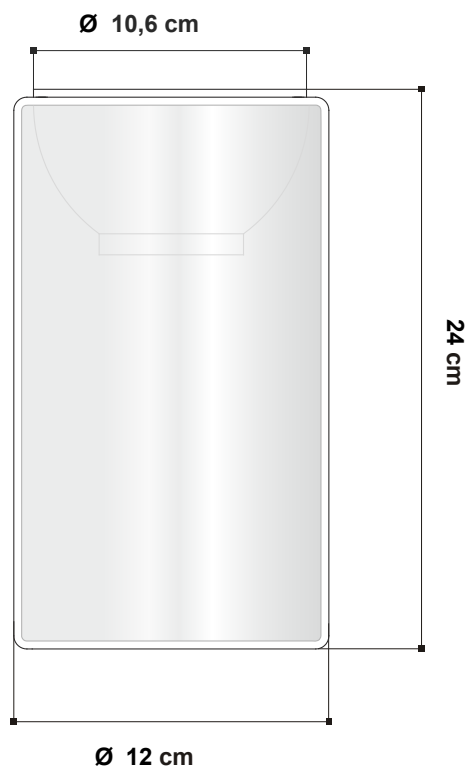
Dimensioni - Dimensions
