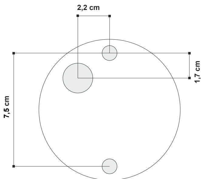
Schema di fissaggio a plafone Outline for ceiling fitting
