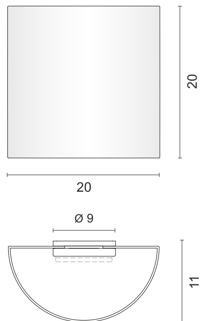
Dimensioni - Dimensions
