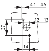
Drilling dimensions door
