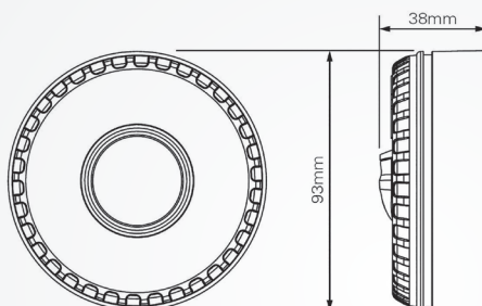
Ceiling VAD
