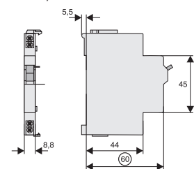
Example: ZP-IHK/(ZP-WHK)+LS
