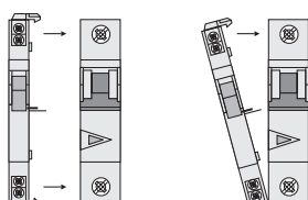
Example: ZP-IHK/(ZP-WHK)+LS
