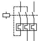
Abbildung 4: Verdrahtung des Motorschutzschalters für den Schutz von Wechselstrom- oder Gleichstrommotoren (Reihenschaltung der Bimetallauslöser)
