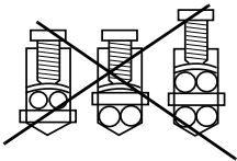
Abbildung 9: Unzulässige Leiteranordnung
