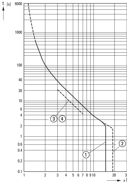
Abbildung/Figure 14: PKZM4-40/XTPR040DC1
