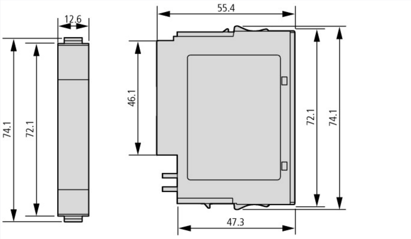
Dimensioni
