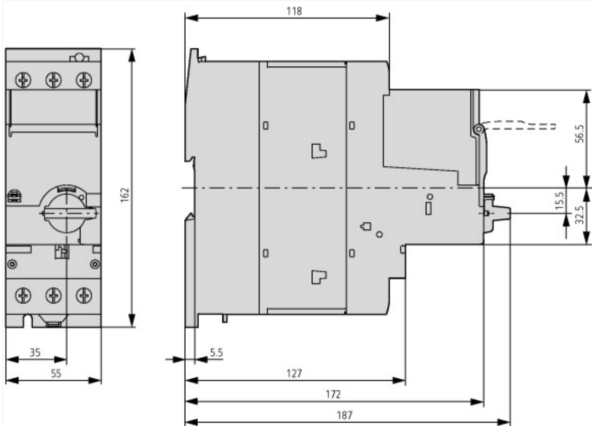
Apparecchio base con unità di sgancio
