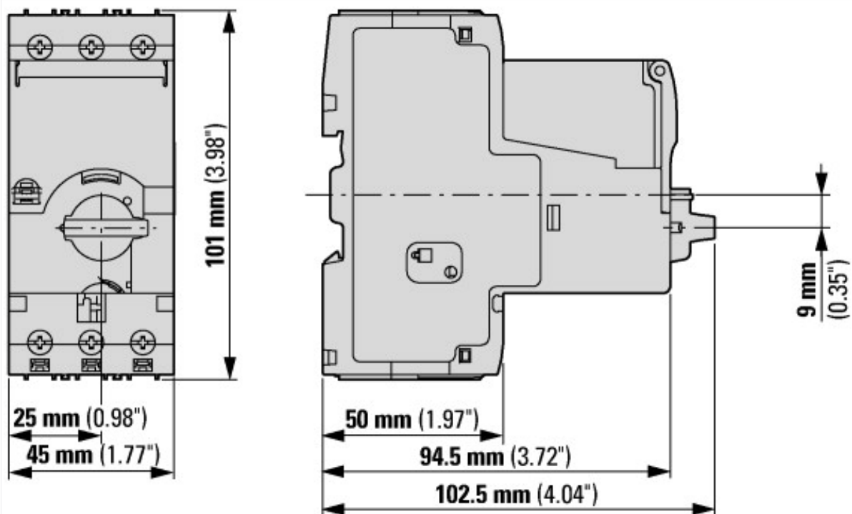
Apparecchio base con unità di sgancio
