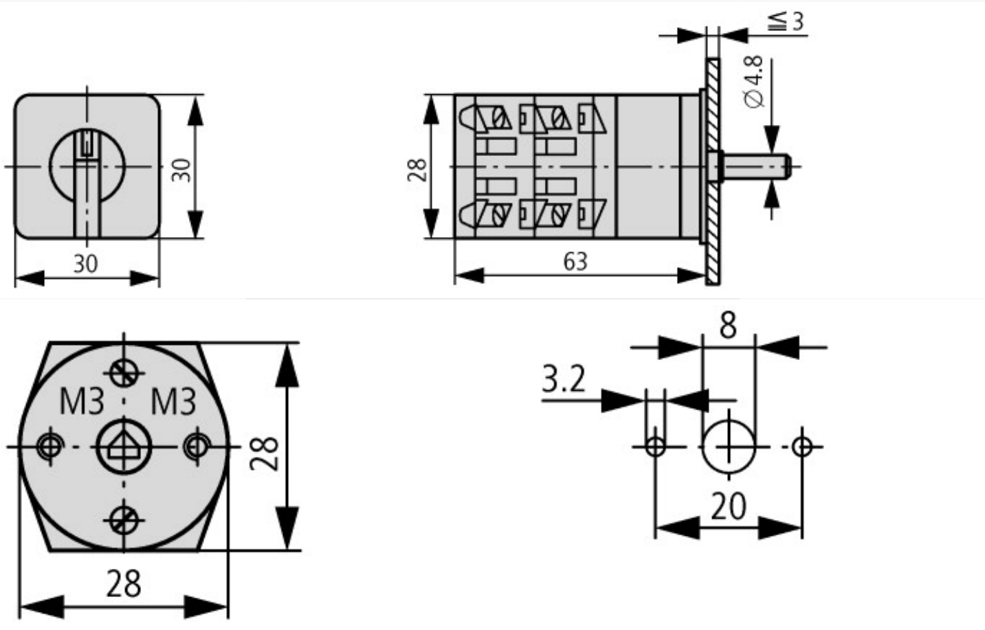
Foratura antina
