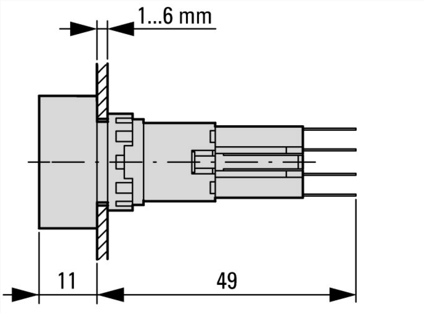
Elementi di azionamento e segnalazione Esecuzione quadrata
