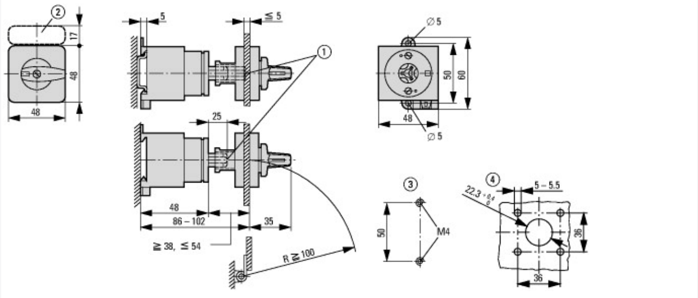
① Prolungamento asse possibile con ZAV-T0, max. 4 x 25 = 100 mm
