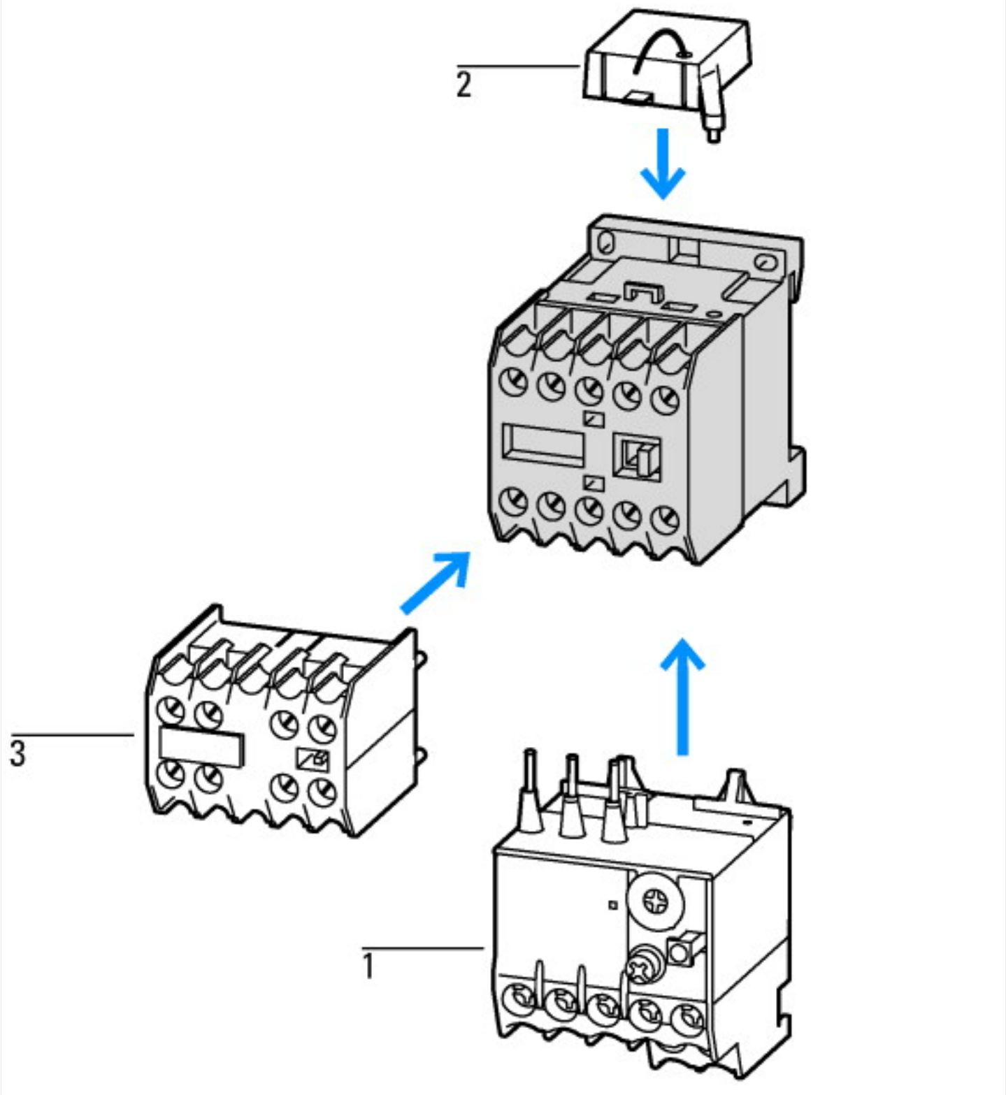
1: Relè termici 2: Circuito di protezione 3: Moduli contatti ausiliari Custodia ad isolamento totale
