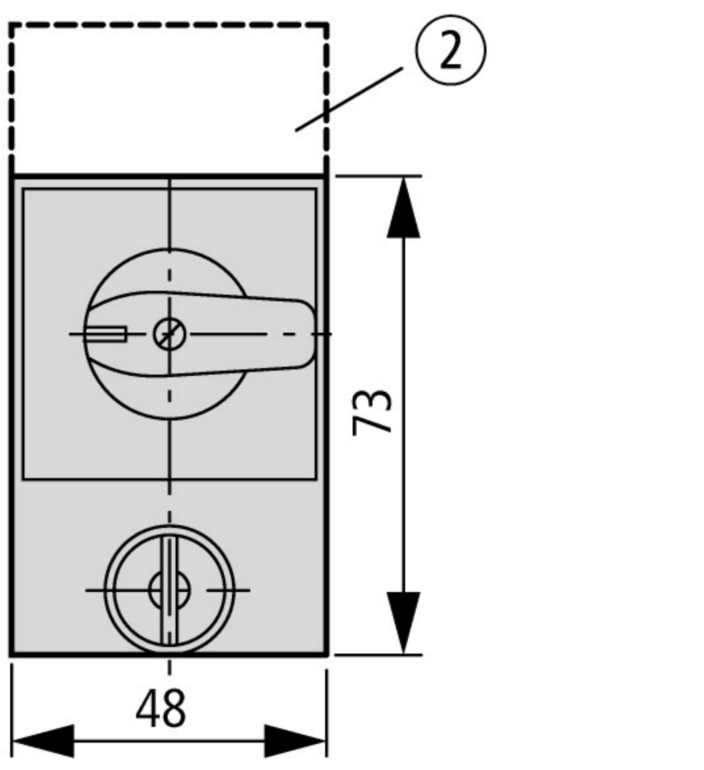
SVA-T3 ② Piastra di supporto ZFS-... non compresa nella fornitura
