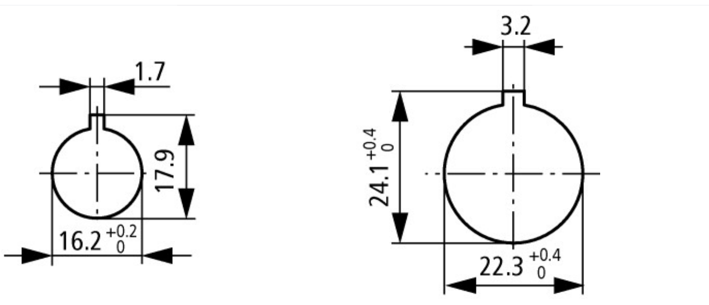
Foratura antenna Fori facoltativi: 16,2 mm = senza riduzione Δ RMQ16; 22,3 mm = con riduzione Δ RMQ-Titan
