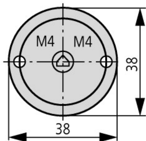
Foratura antina
