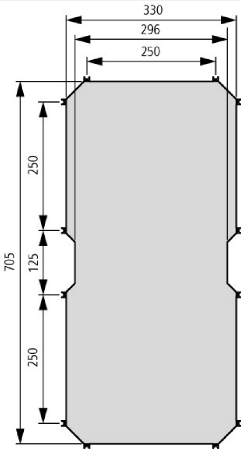
Piastra di montaggio M3-....: spessore 3 mm
