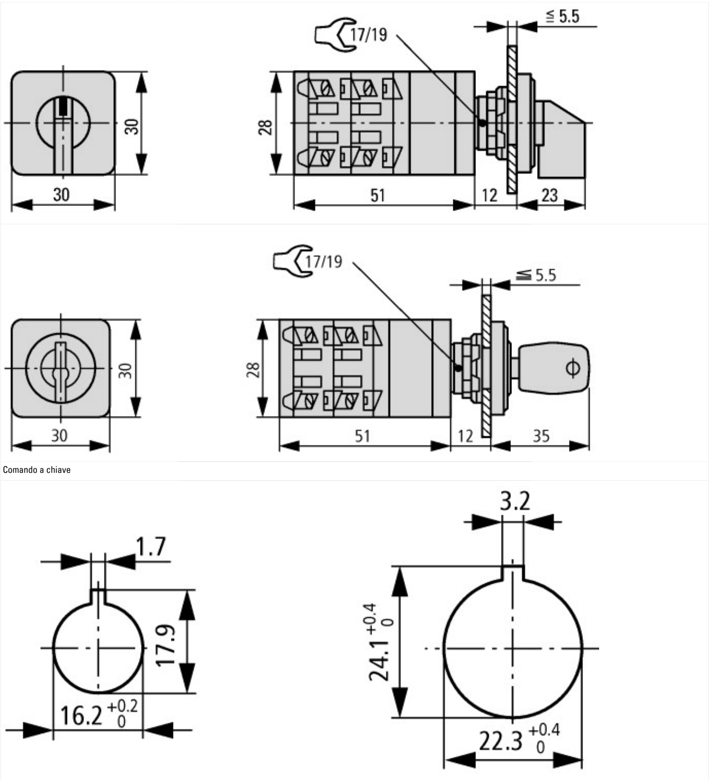
Foratura antenna Fori facoltativi: 16,2 mm = senza riduzione \triangle RMQ16; 22,3 mm = con riduzione \triangle RMQ-Titan
