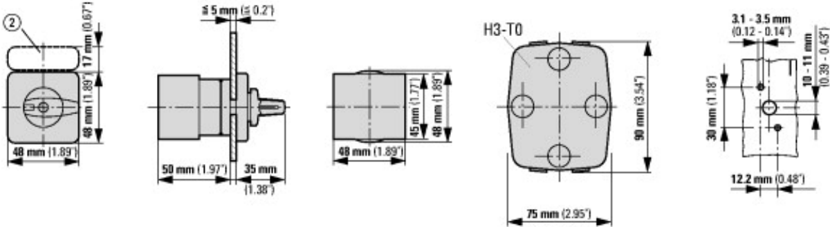
② Piastra di supporto ZFS-... non compresa nella fornitura
