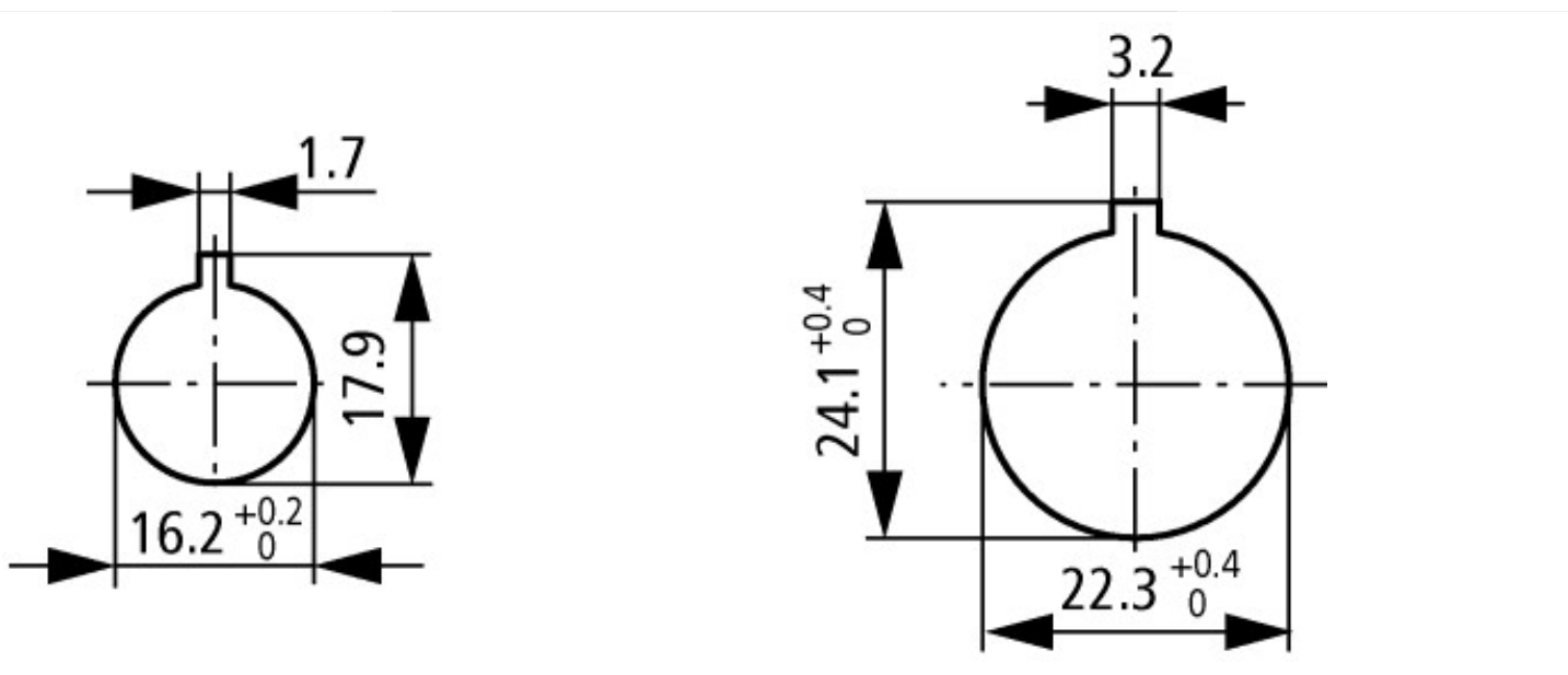
Foratura antina Fori facoltativi: 16,2 mm = senza riduzione ± RMQ16; 22,3 mm = con riduzione ± RMQ-Titan
