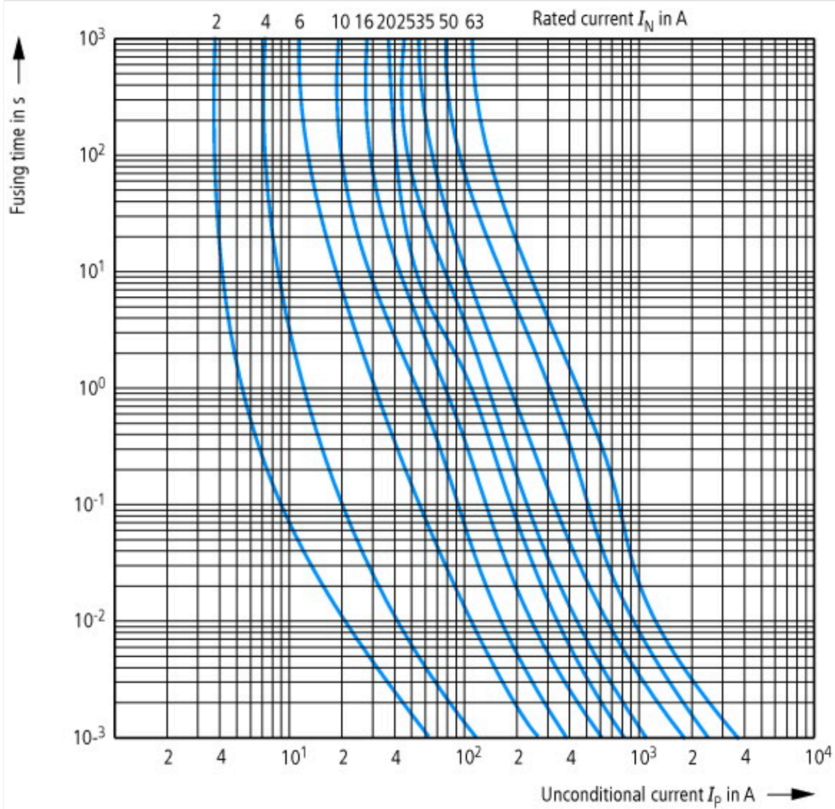
Linea caratteristica tempo-corrente fusibili D0 2...63 A gG(gL)
