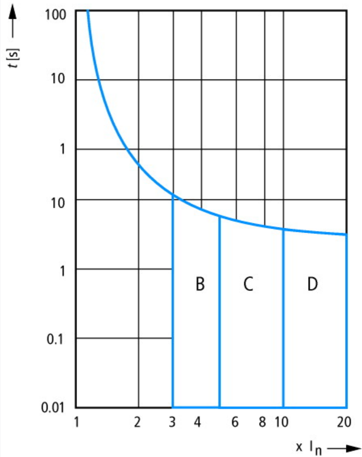
Caratteristiche dell'intervento FAX a 30 °C: B, C, D conforme a IEC/EN 60898
