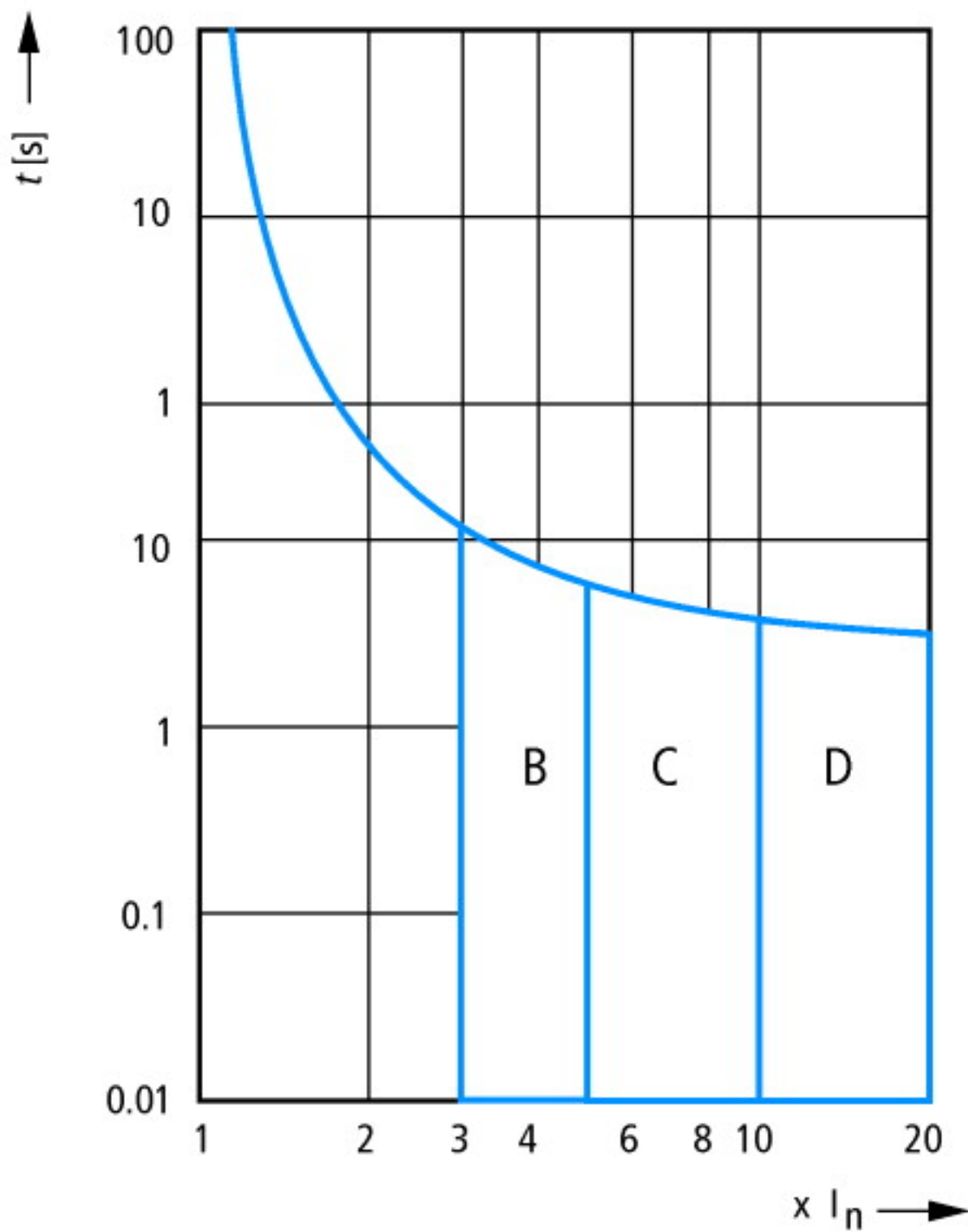
Curva caratteristica d'intervento FAZ a 30°C B, C, D secondo IEC/EN 60898
