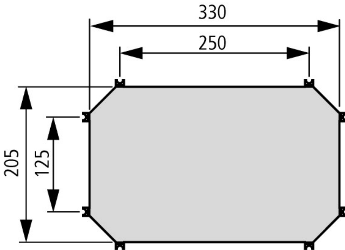
Piastra di montaggio MM-CL...: Spessore 1,5 mm
