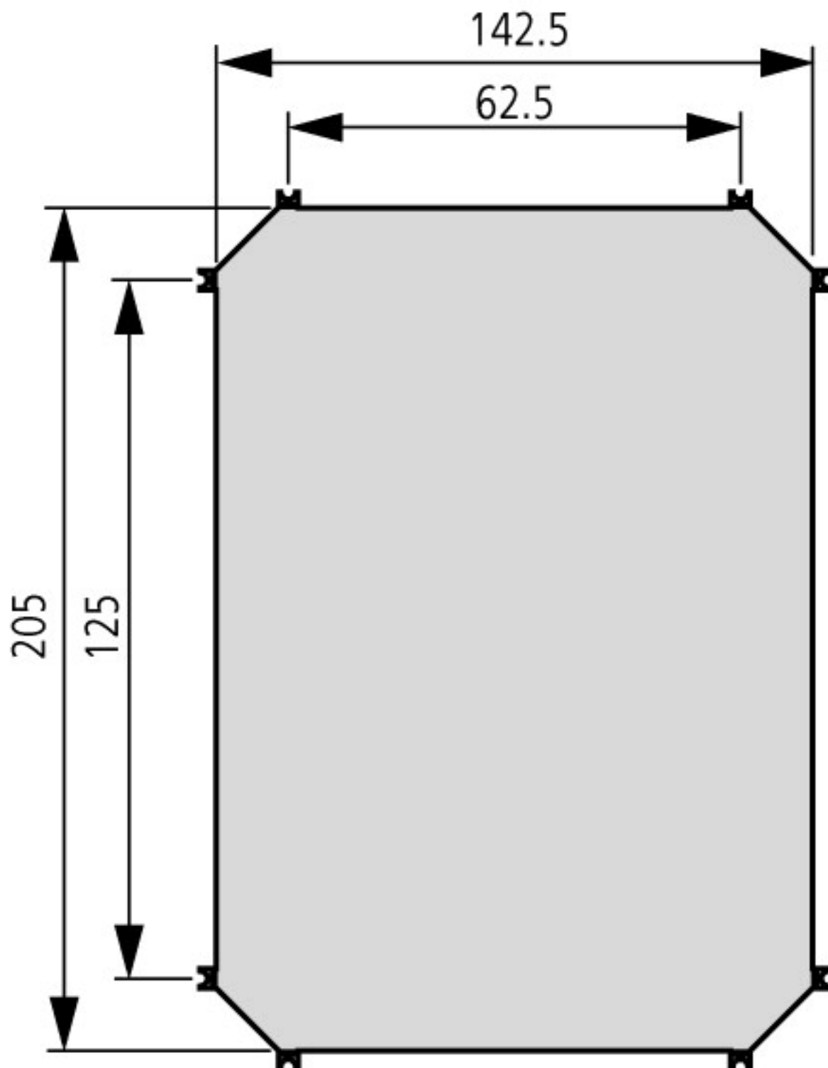
Piastra di montaggio MM-CL...: Spessore 1,5 mm
