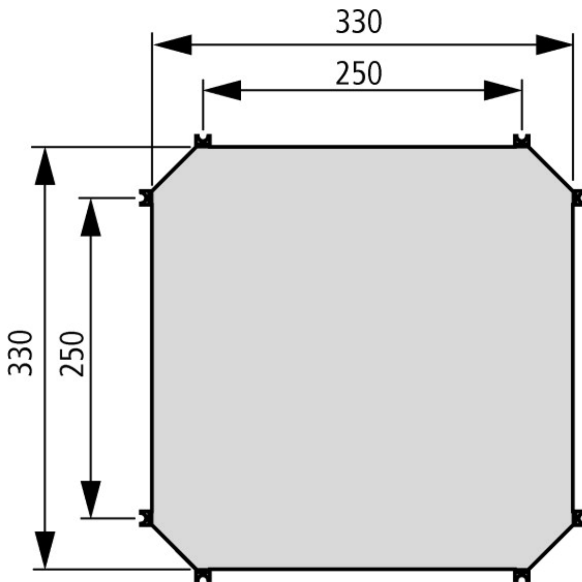
Piastra di montaggio M-Cl...: Spessore 2 mm
