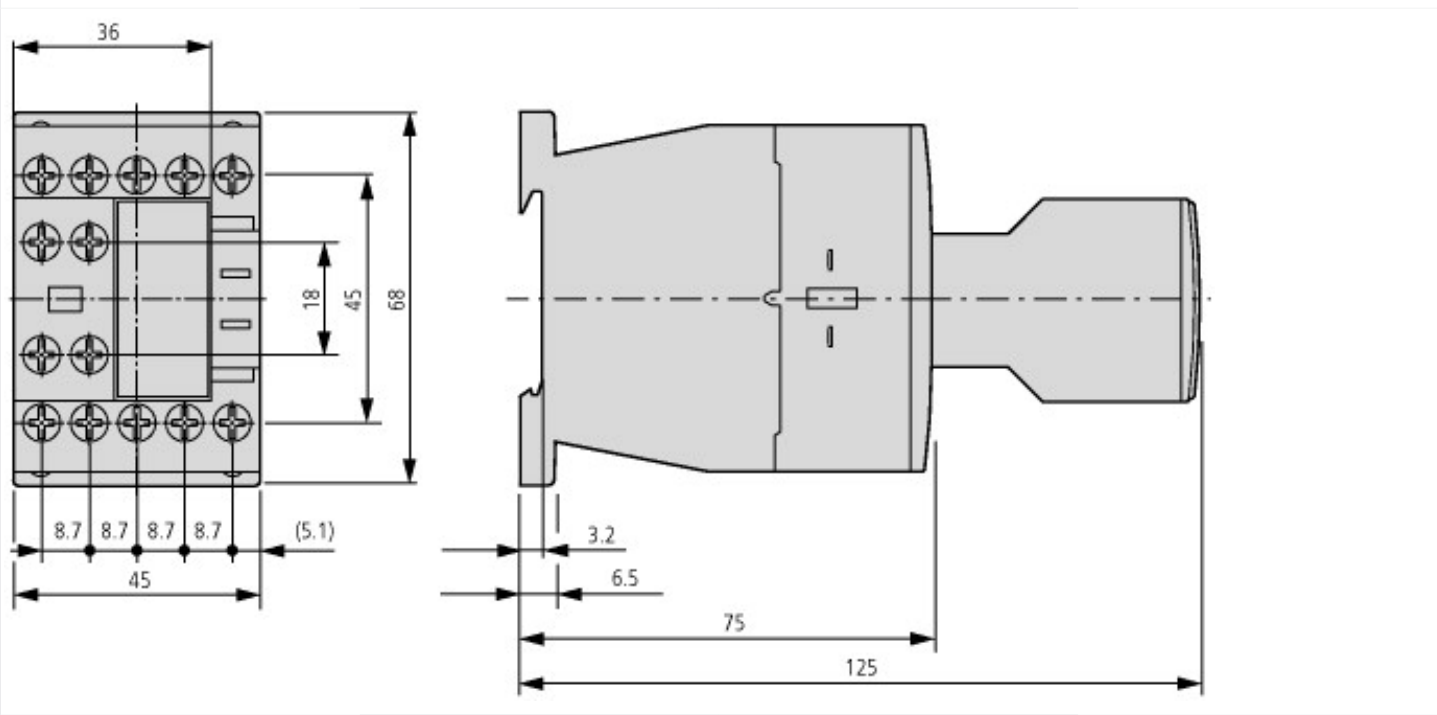
contattore di potenza con modulo contatti ausiliari DILA-XHIT...
